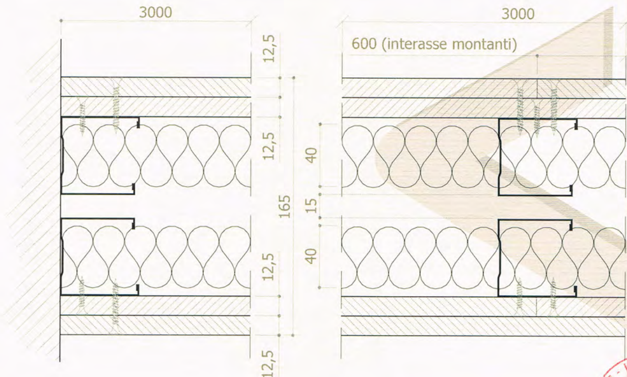
Particolare sezione orizzontale
