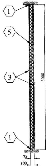
Sezione B:B
