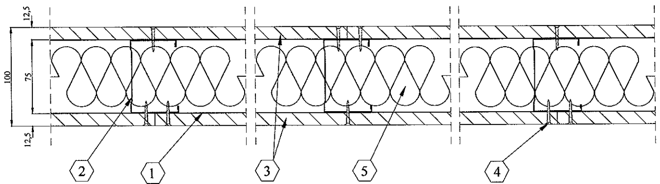
Sezione A:A
