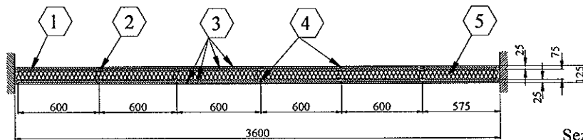
Sezione B:B
