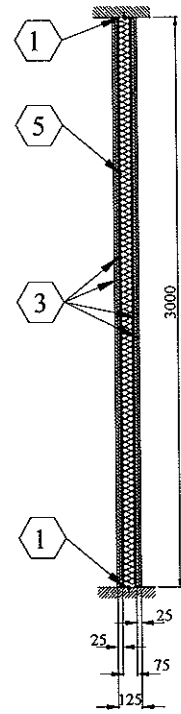
Sezione B:B
