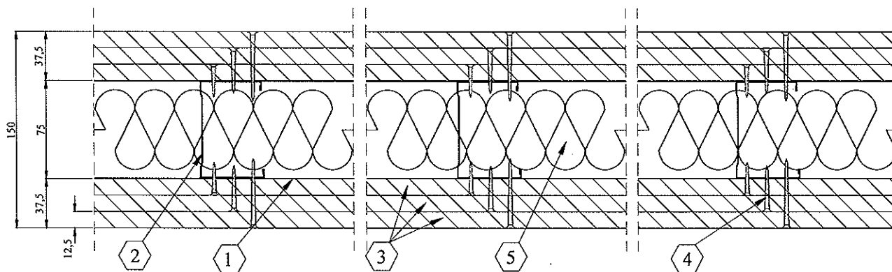
Sezione A:A
