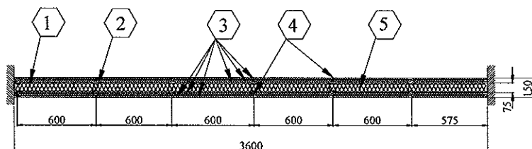
Sezione A:A
