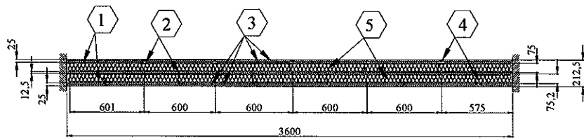
Sezione A:A
