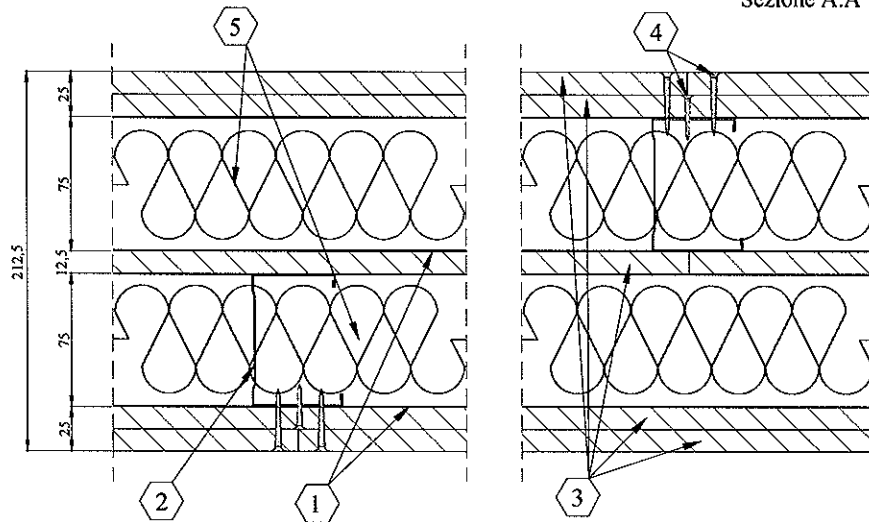
Sezione A:A
